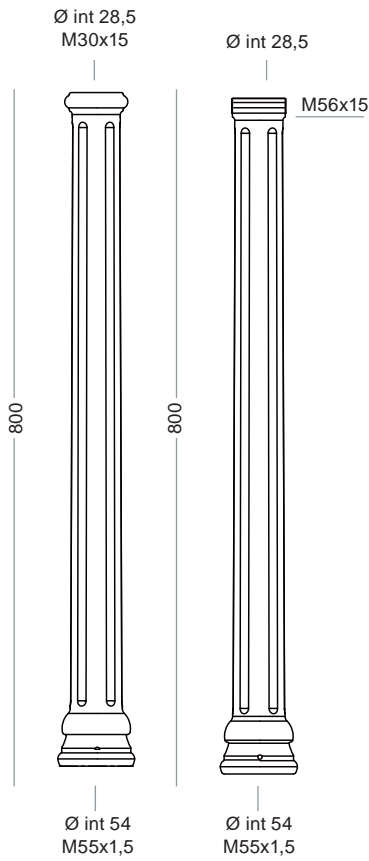
6047-A Prolunga - Joint Optional
