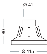
6017-A Per tubo Ø 45 For tube Ø 45
