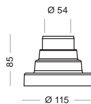
6015-A Tornita Ø est. 54 per tubo Ø 60 Tuorned ext. Ø 54 for tube Ø 60
