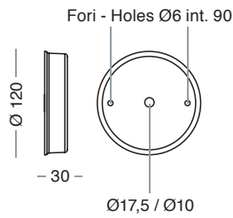
1302-A Foro - Hole \varnothing 17,5 1302-A-1 Foro - Hole \varnothing 10
