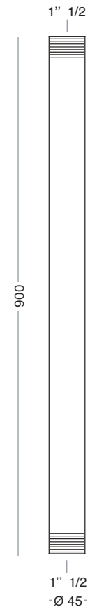
8165-A Tubo per fissaggio ferro zincato Fixing tube zincate iron
