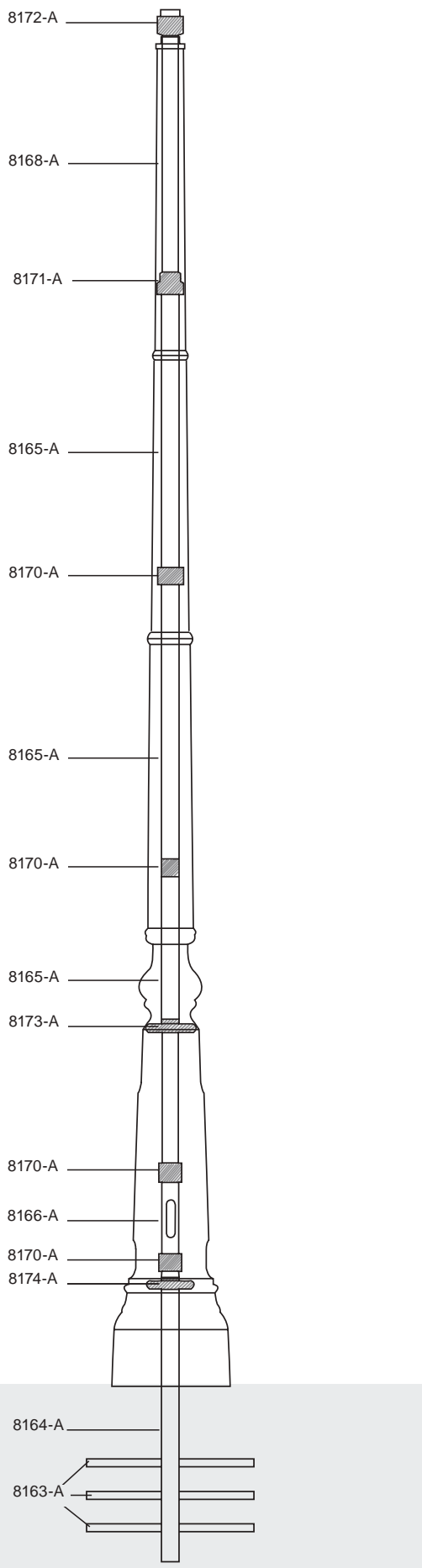
Struttura interna Palo - Internal pole structure
