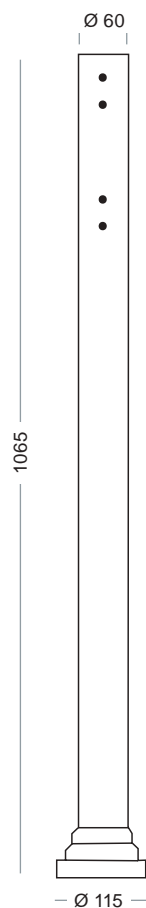
6095-A-1 1 luce - 1 light 6095-A 1mt
