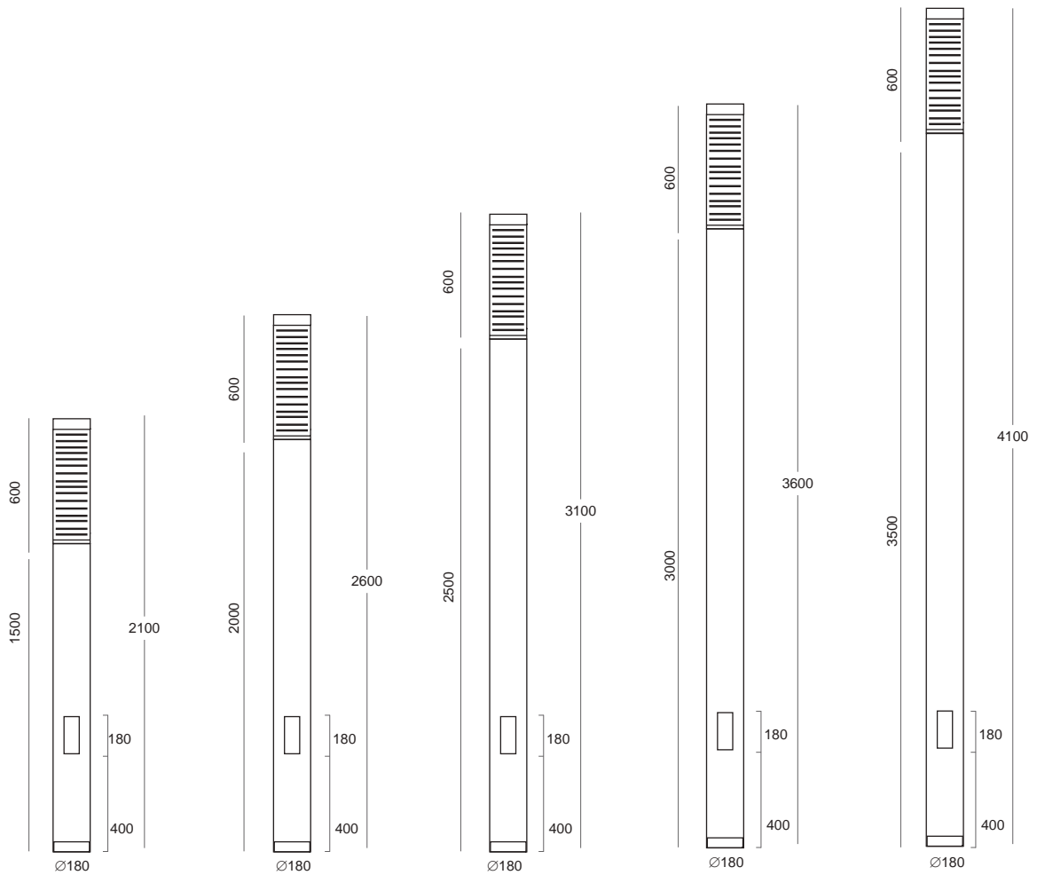
F1273-13-011 Kit unità elettrica - Electric unit kit 2G11
