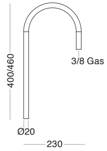
1600-A H400 x L230 1610-A H460 x L230
