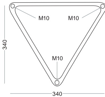
5013-A Dima di fissaggio per base 6040-A Fixing accessory for base 6040-A
