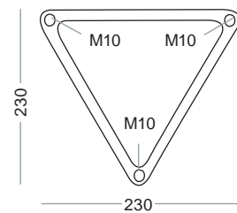
5014-A Dima di fissaggio per base 6041-A - 6032-A - 6058-A Fixing accessory for base 6041-A - 6032-A - 6058-A
