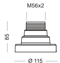
6015-A-1 Filetto M56x2 Thread M56x2
