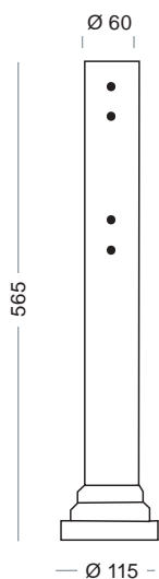
6094-A-1 1 luce - 1 light 6094-A 0,50mt
