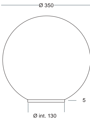
7456-A PC Trasparente - Transparent PC 7456-A-O PC Opale - Opal PC
