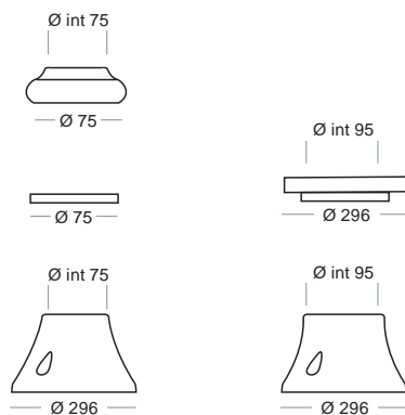
6222-A H 2505 Ø 75 6218-A H 3200 Ø 75 6219-A H 4300 Ø 75
