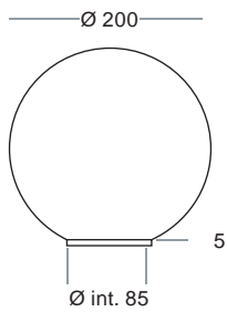
7451-A PC Trasparente - Transparent PC 7451-A-O PC Opale - Opal PC
