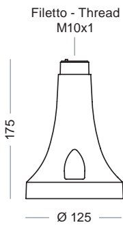
11611-A *Box 7195-A pag. 293 Base - Base
