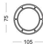
7005-A Nylon Adattatore tra 6004-A-1 e 6005-A Adapter between 6004-A-1 and 6005-A
