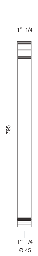
8168-A Tubo per fissaggio ferro zincato Fixing tube zincate iron
