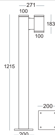
13024-A Palo per 204
