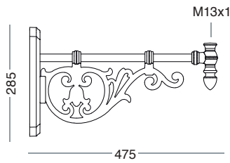
1068-A Fissaggio a muro - Wall fixing
