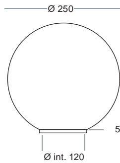
7452-A PC Trasparente - Transparent PC 7452-A-O PC Opale - Opal PC
