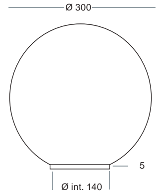
7453-A PC Trasparente - Transparent PC 7453-A-O PC Opale - Opal PC
