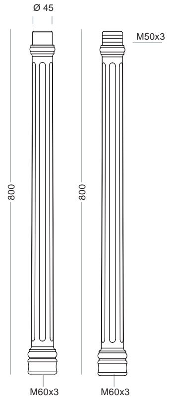
6048-A-1 Palo sopra - Upper pole
