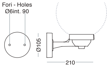
1006-A Per globo - For globo Ø200
