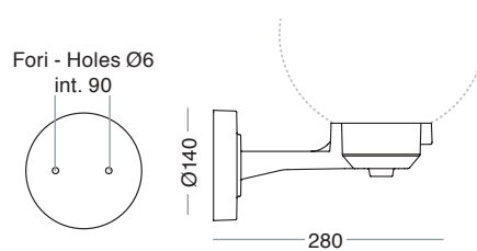
1007-A Per globo - For globo Ø250
