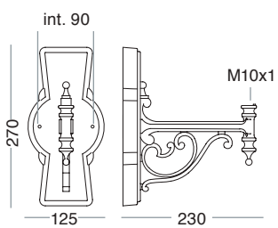
1005-A *Kit 7195-A pag. 29
