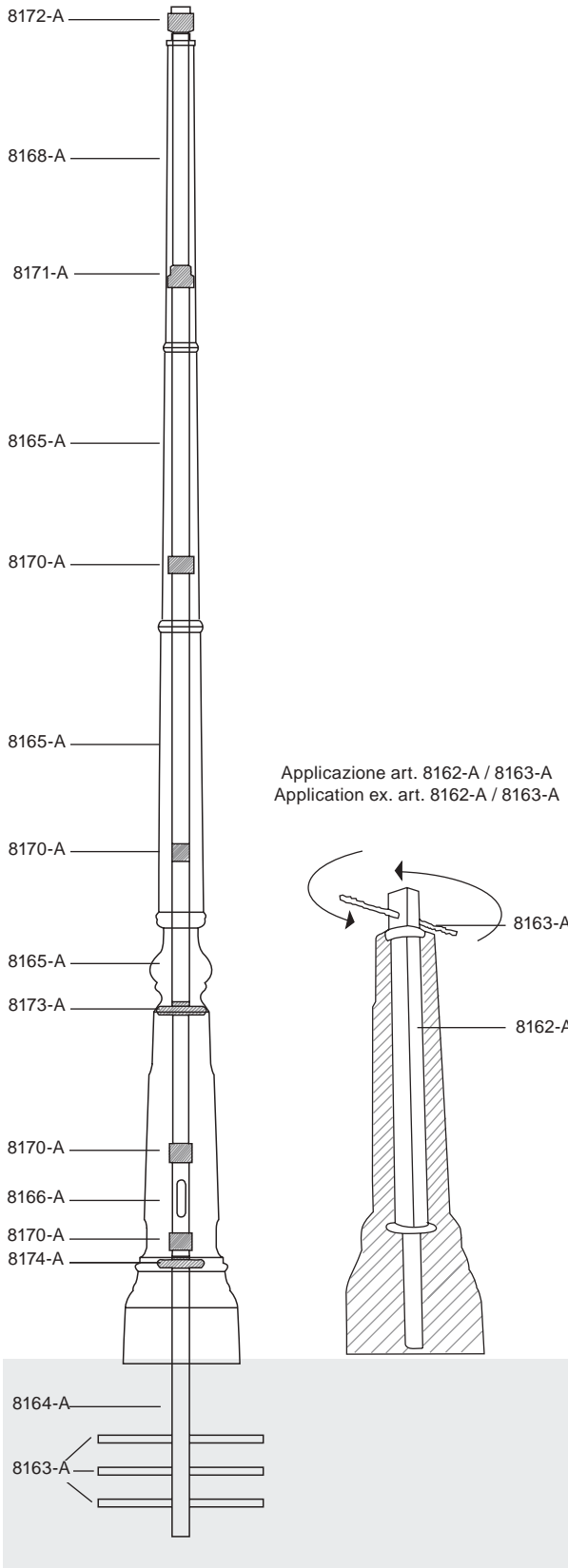
Struttura interna Palo - Internal pole structure
