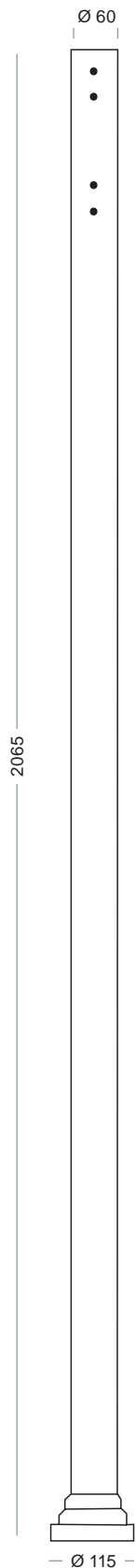
6097-A-3 3 luci - 3 lights 6097-A-2 2 luci - 2 lights 6097-A-1 1 luce - 1 light 6097-A 2mt
