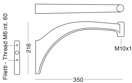
1046-A-1 Fissaggio a muro - Wall fixing
