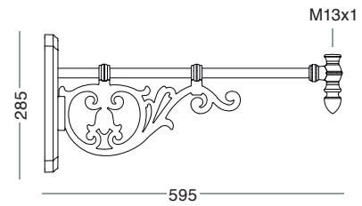
1069-A Fissaggio a muro - Wall fixing
